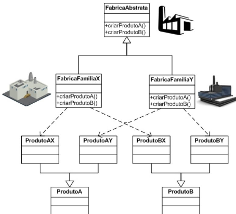
Figura 6.2: Estrutura Básica do Abstract Factory
