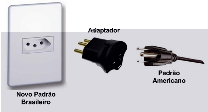
Figura 5.5: Representação do adaptador de tomadas
