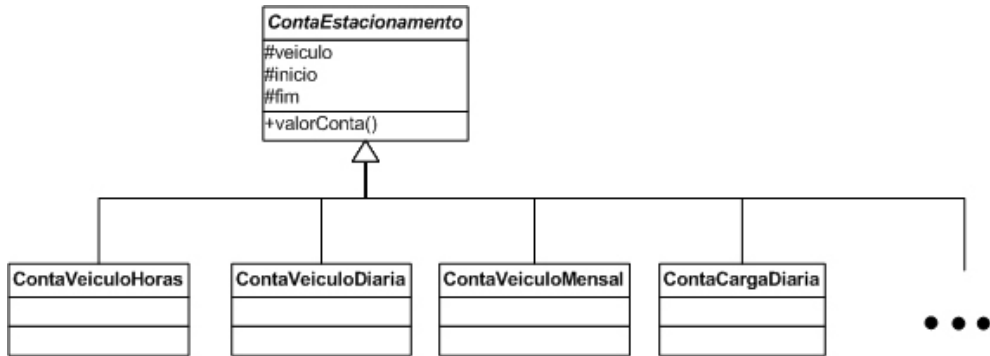
Figura 1.1: Utilização de herança para dividir a lógica
