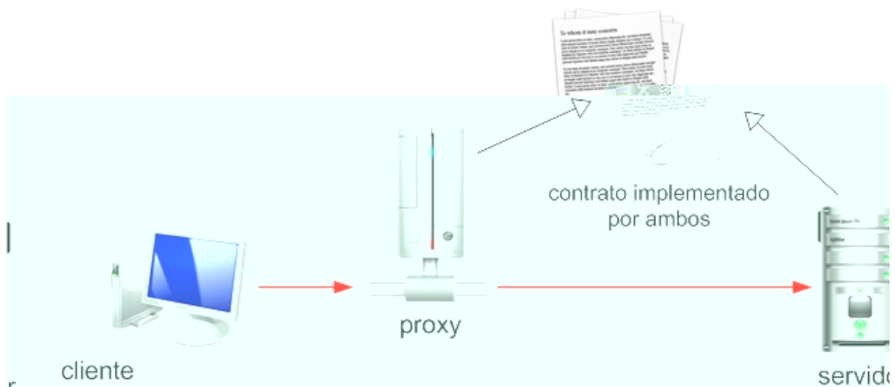
Figura 10.2: Estrutura de um Proxy para Criação de Arquitetura
