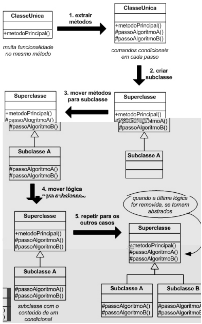
Figura 2.4: Quebrando classe única com método grande e complexo
