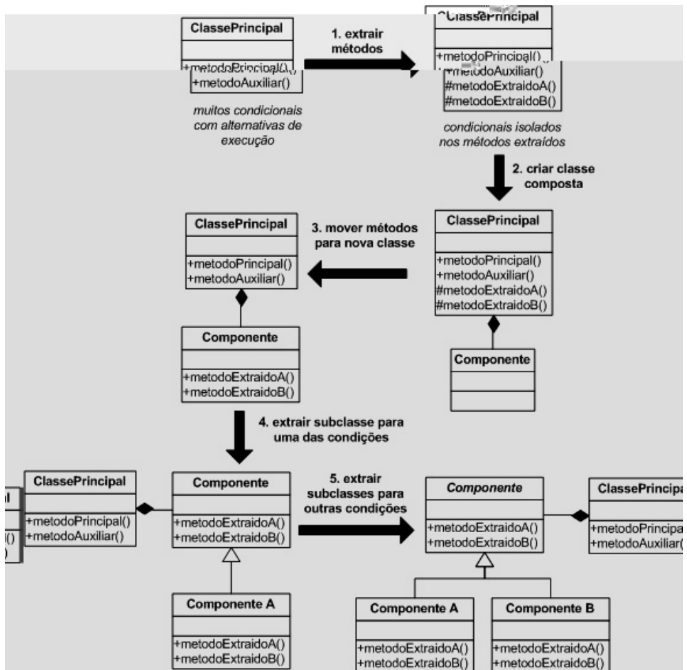
Figura 3.8: Refatorando em Direção a Composição
