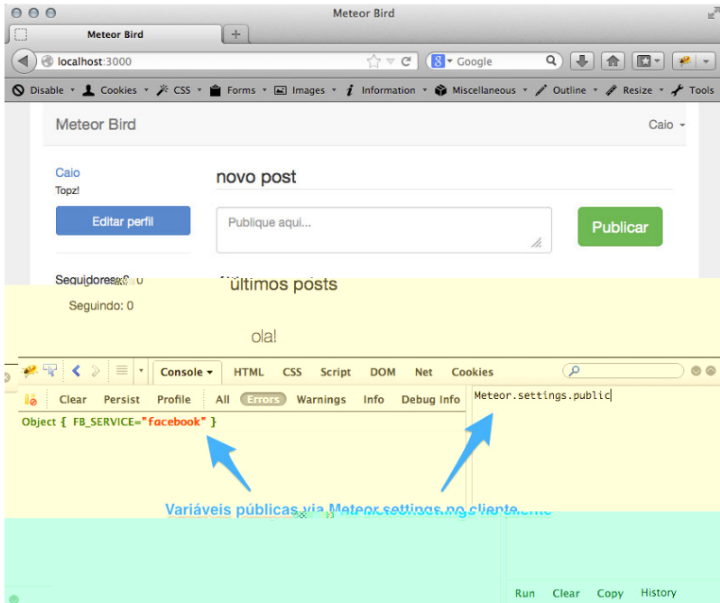
Figura 1.1 : Usando Meteor.settings no cliente.
