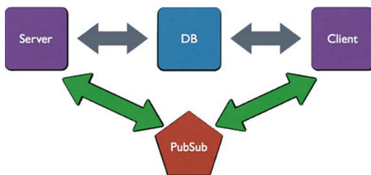
Figura . : Banco de dados compartilhado entre cliente e servidor.
