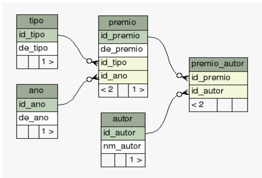
Fig. . : Modelo relacional dos ganhadores
