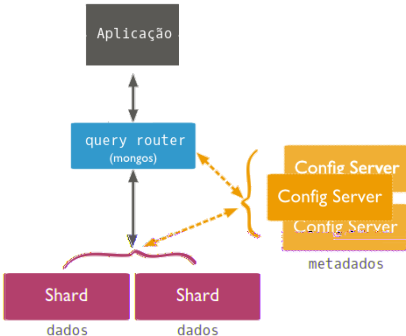
Fig. 1.1 : MongoDB com particionamento (sharding)
