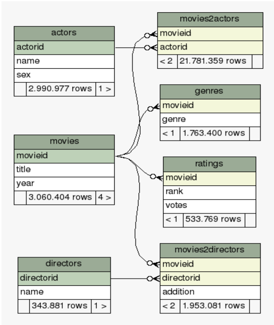
Fig. . : Modelo relacional de meus filmes
