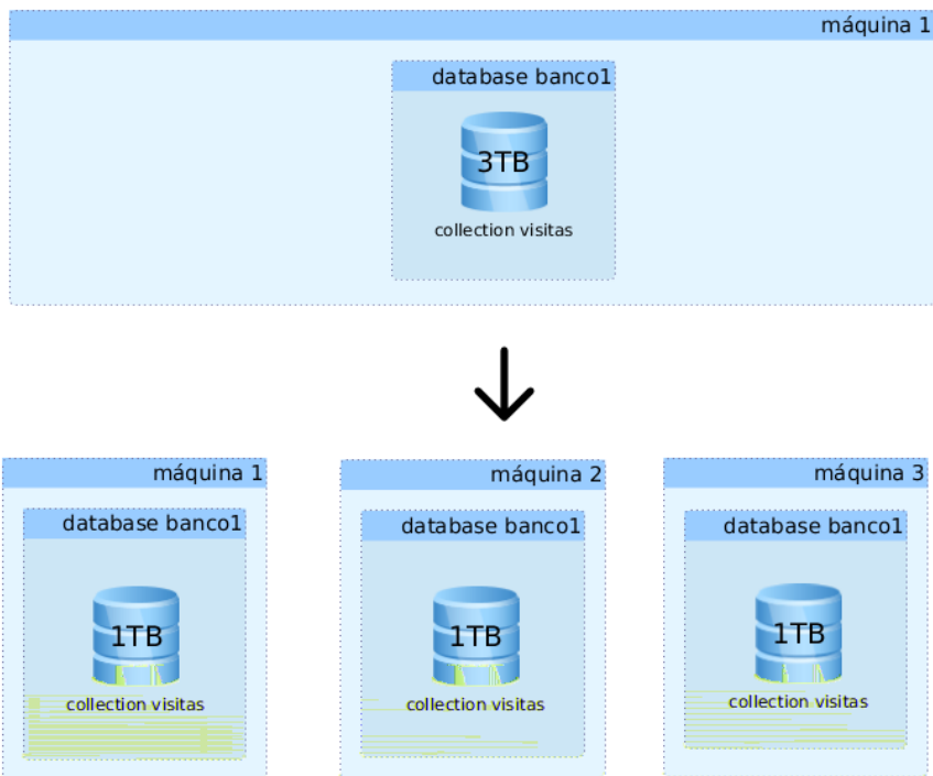
Fig. 10.1 : Sharding
