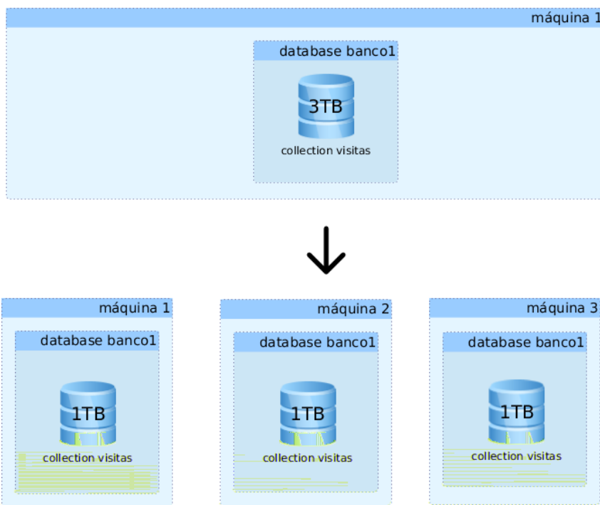
Fig. . : Sharding
