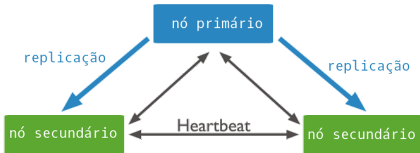
Fig. . . : MongoDB replica set com três nós
