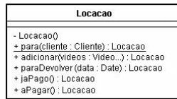
Fig. . : Diagrama de classes
