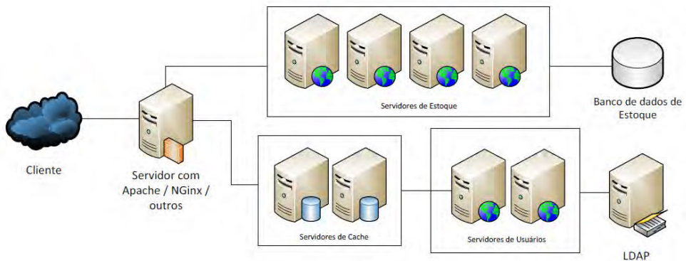
Figura 10.1: Estrutura separada dos serviços
