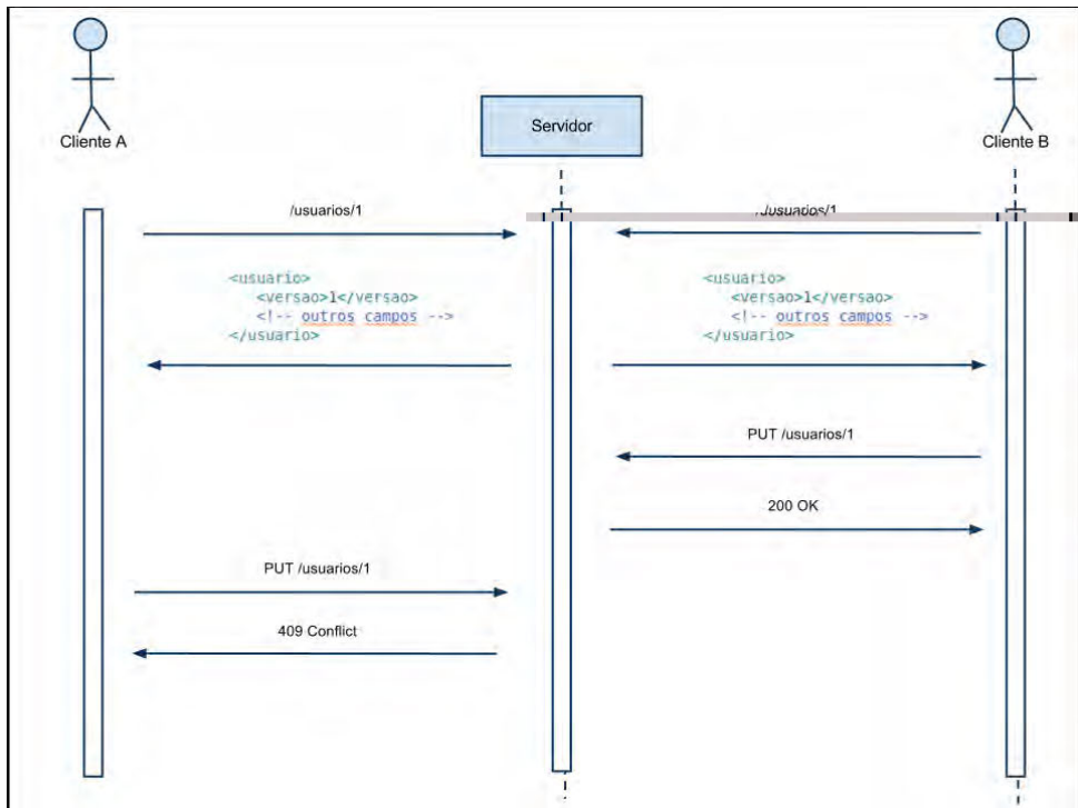
Figura 10.1: Controle de versões com REST
