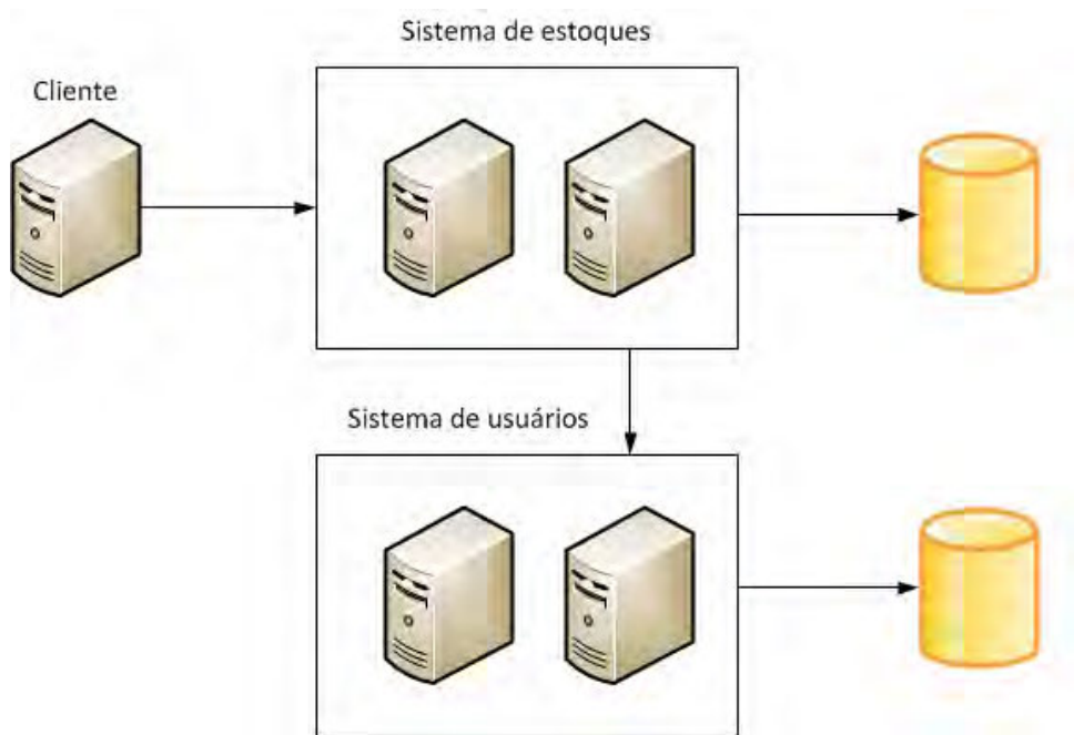
Figura 1.1 : Arquitetura das aplicações knight.com
