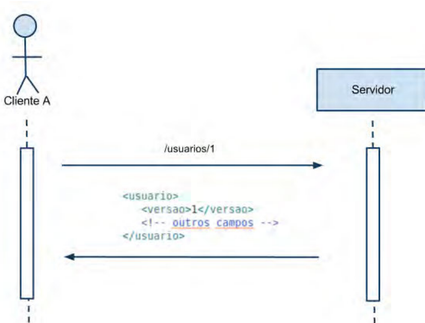
Figura 10 : Solicitação de recurso com versionamento
