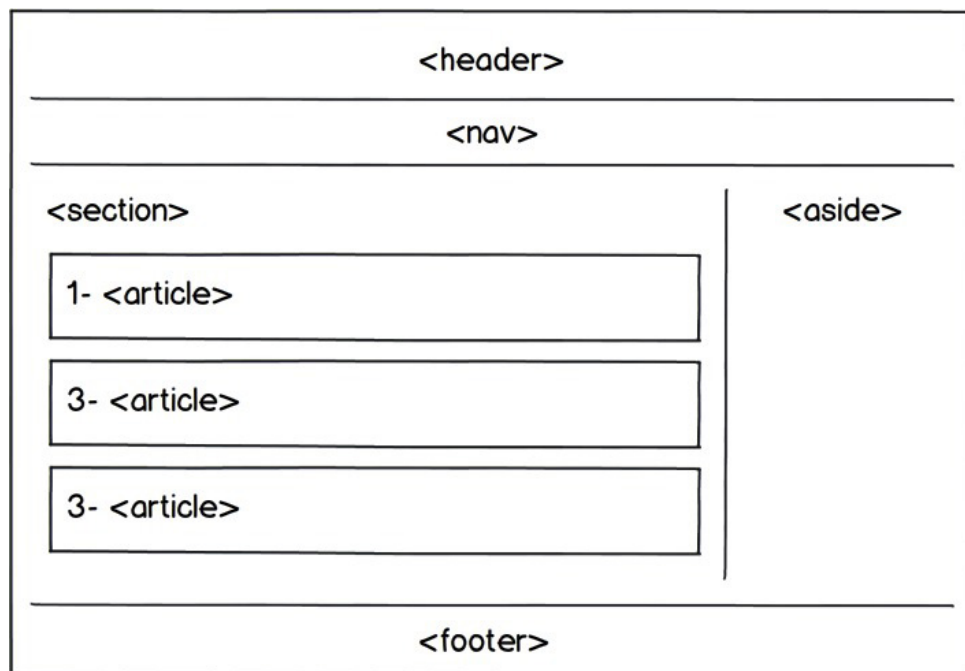
Figura 3.1: O papel de cada elemento novo em uma página completa.
