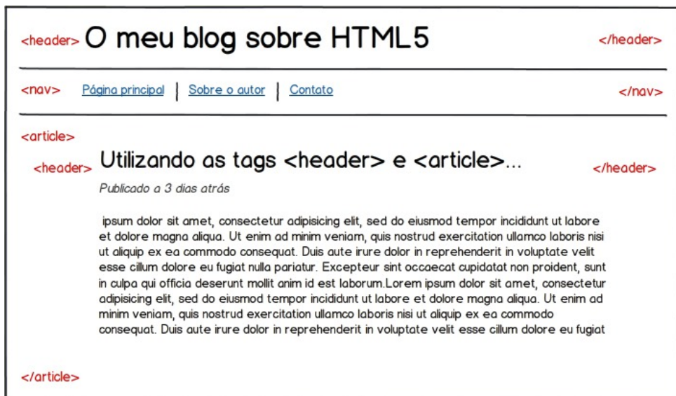
Figura 3.2: Um mockup do exemplo descrito - a tag ' <header> ' pode aparecer em 2 seções diferentes.
